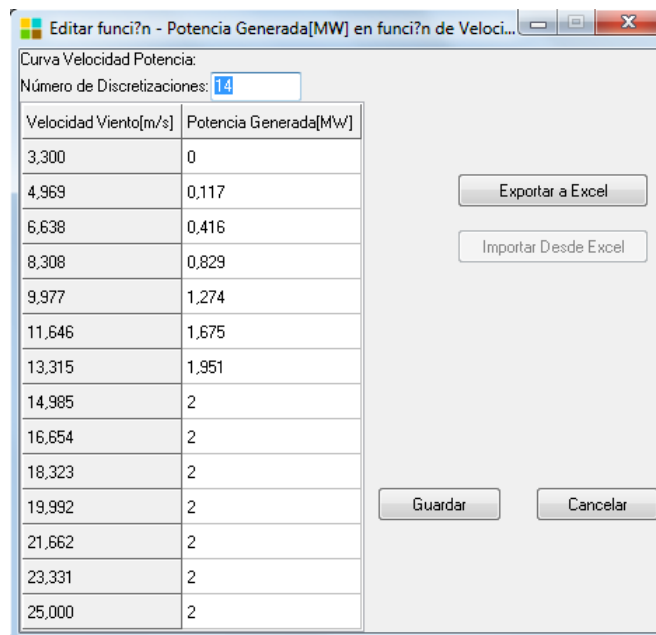
Fig. 19: Editor Curva Velocidad-Potencia.
