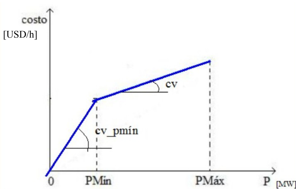
Fig. 28: Costo de producción de una central térmica con mínimo técnico.
